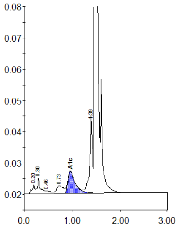
Peak table - ID: 10004608
