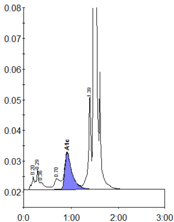
Peak table - ID: 10013779
