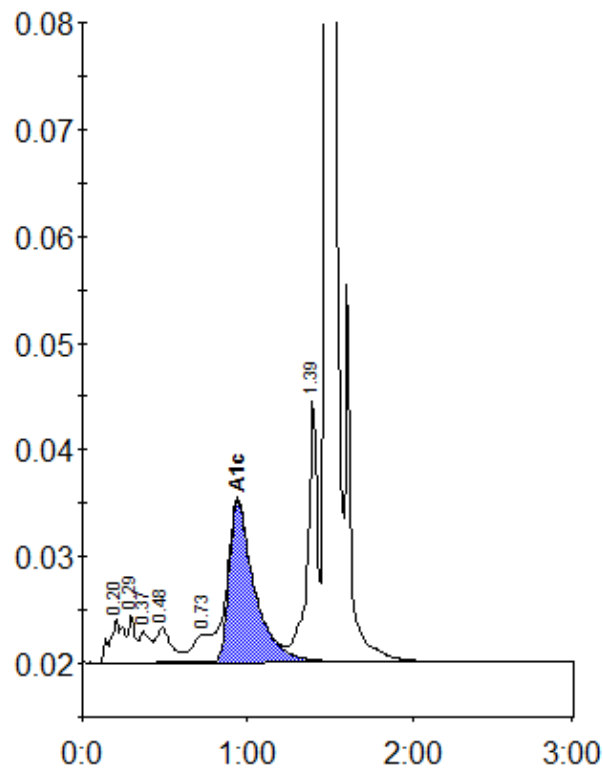
Peak table - ID: 10018117
