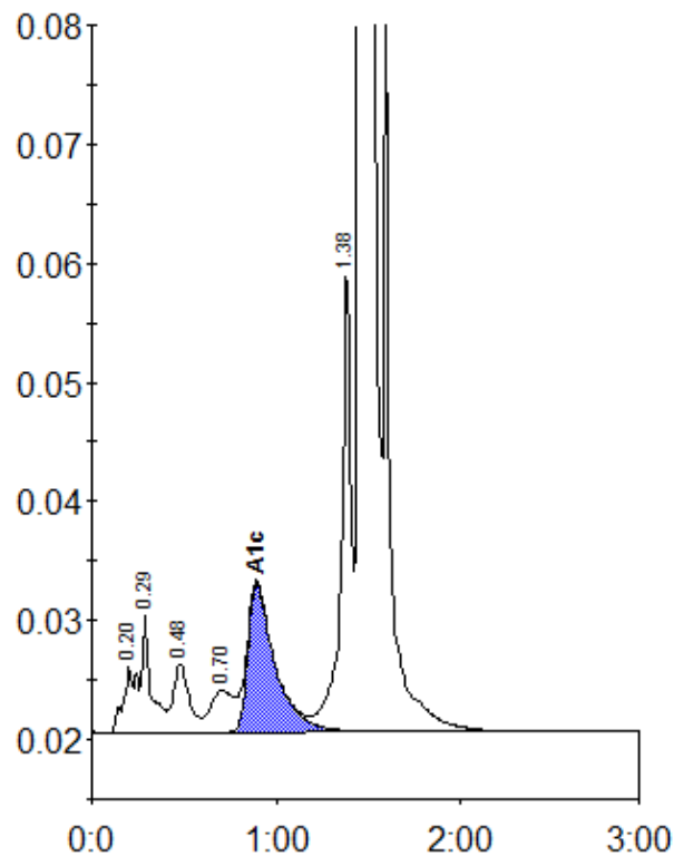
Peak table - ID: 10019279
