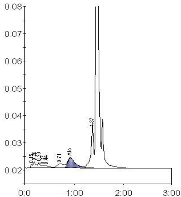
Peak table - ID: 10020828
