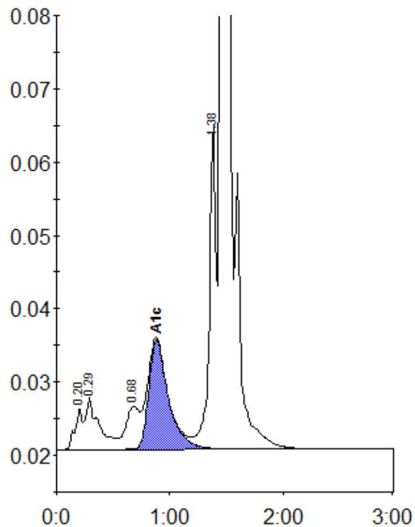
Peak table - ID: 10032659
