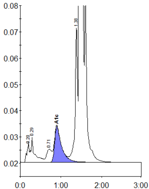
Peak table - ID: 10051134
