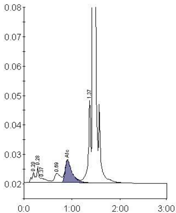
Peak table - ID: 10056549
