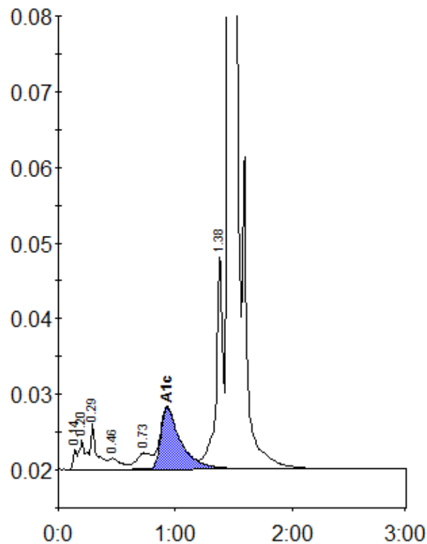
Peak table - ID: 10074619
