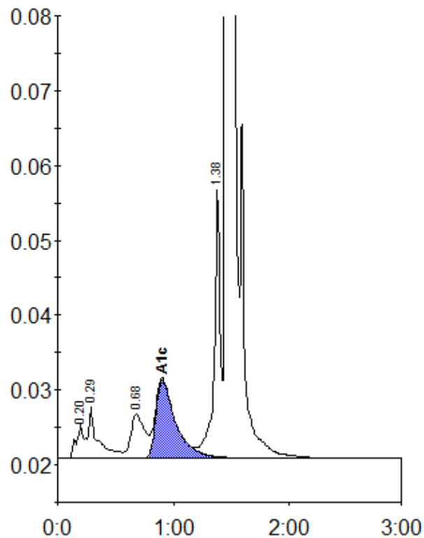
Peak table - ID: 10076263
